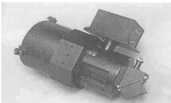
Fig. 1-10. Basic OCD unit.
