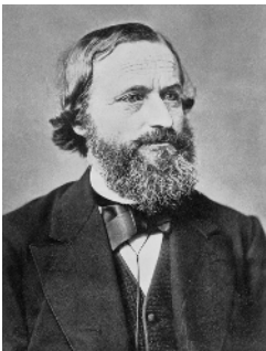
Gustav Kirchhoff (1824–1887)
