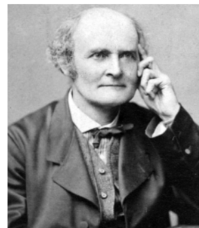
Arthur Cayley (1821–1895)
