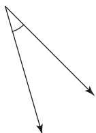
Acute angle
